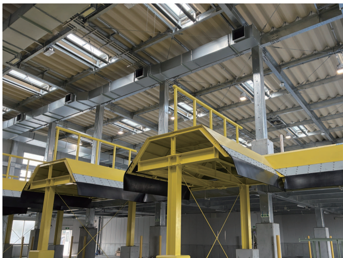
1階搬出スペース（ごみ受入口）
